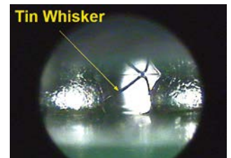
PBGA: tin whisker
