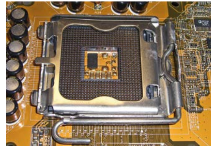
LGA 775-Prozessorsocket
