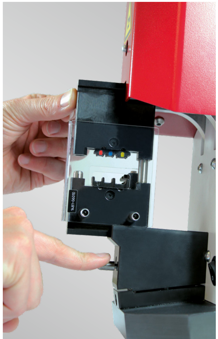
Einfaches Austauschen der Adapter Easy exchange of adapters
